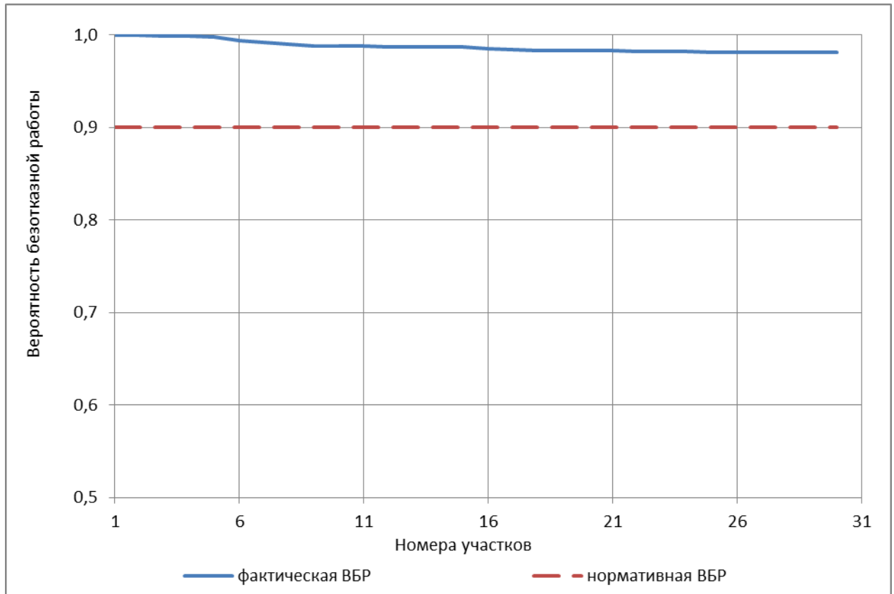
Рисунок 3.65 – ВБР относительно ТК конечного потребителя «ПТ-Замкнут,15 эЗ» теплопроводов зоны котельной АО «Теплоэнерго» по пр. Союзный, д. 43 (расчетный путь 11-3) к 2030 году
